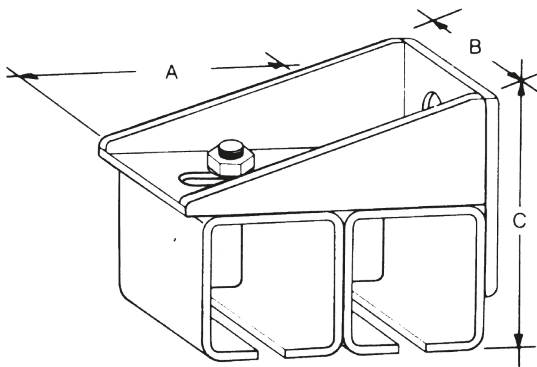
Dobbel veggbrakett
