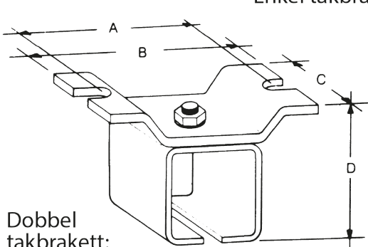
Enkel takbrakett
